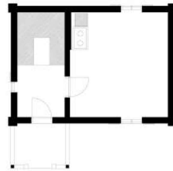
Bild 38. Gårdsbyggnadens planritning.
