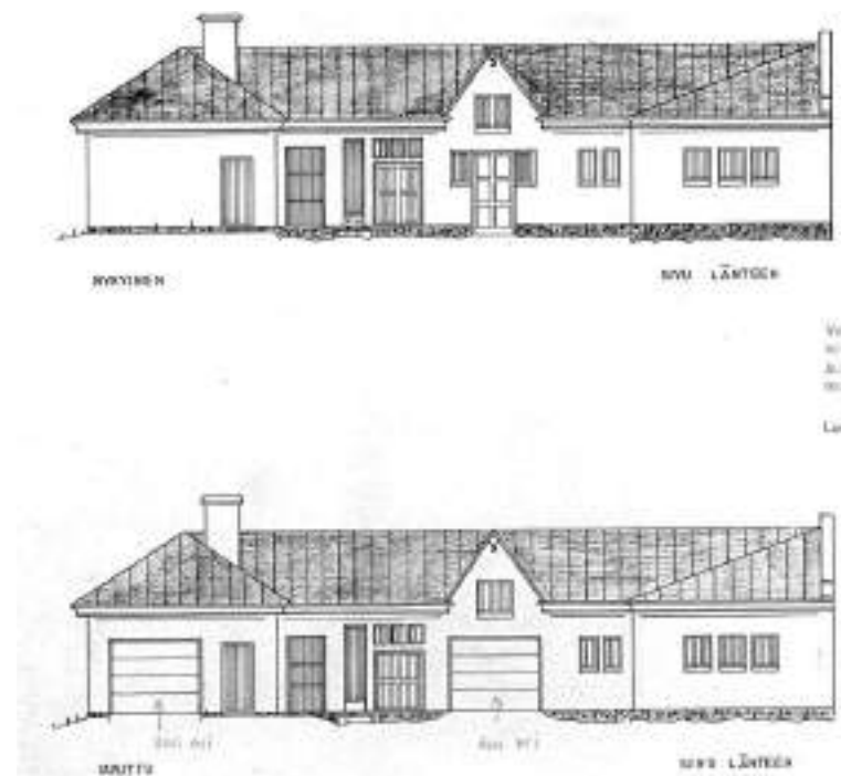
Bild 33. Ändringsritning 1985: 2 garagedörrar, den högra placerad på platsen för ingången till det före detta stallet.
