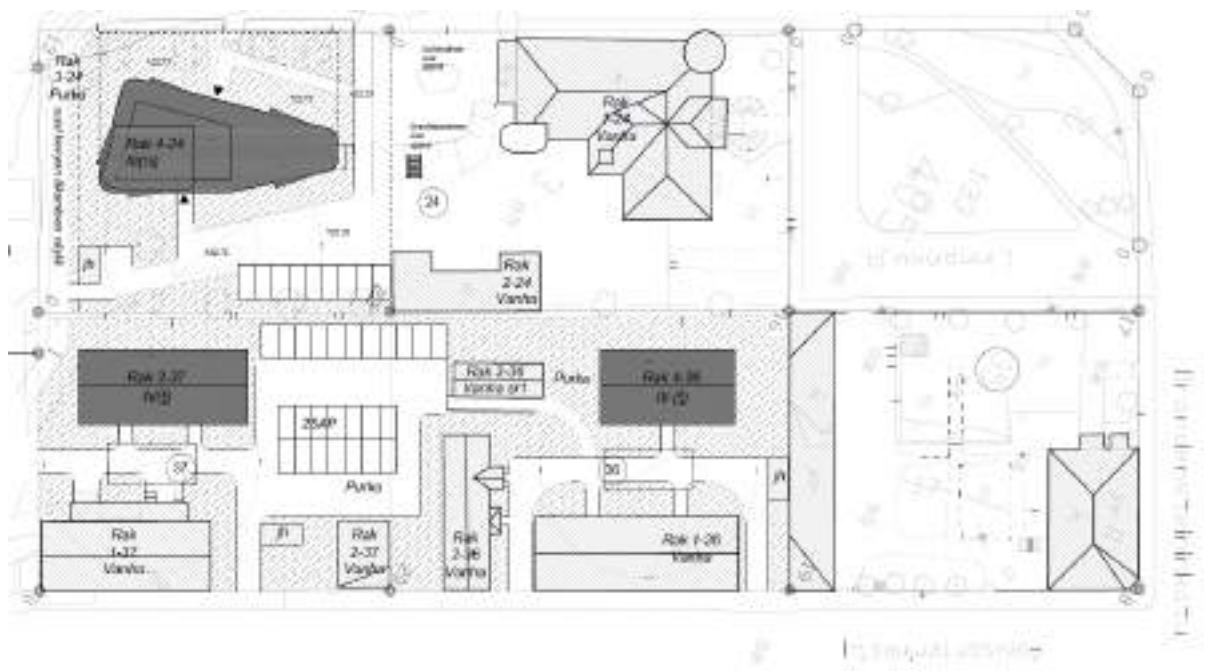
Figur 3-15. Referensplanens situationsplan (Arkkittehtitoimisto Iiro Mikkola 2025)
