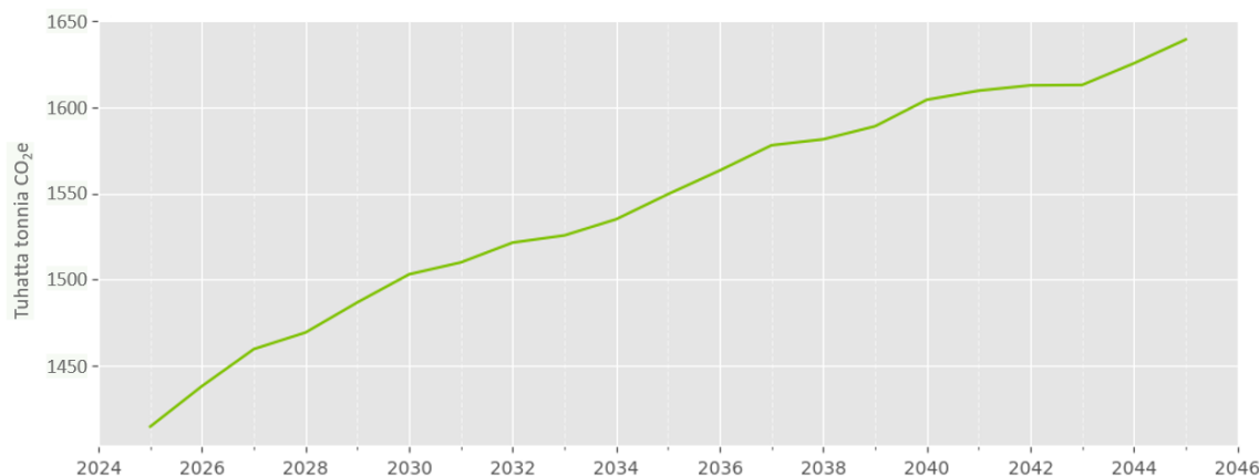
Bild 1: Uppskattad utveckling av Lovisa stads skogars kollager från nuläget till 2045. Mängden kol som lagrats i skogarna ökar jämnt. Uppskattningen innefattar trädbeståndet (levande och dött) samt organiskt kol i markgrunden. Uppskattningen har gjorts i enlighet med antagen skogsskötsel och hyggen, kortfristiga störningar (till exempel stormar) kan medföra avvikelser.
