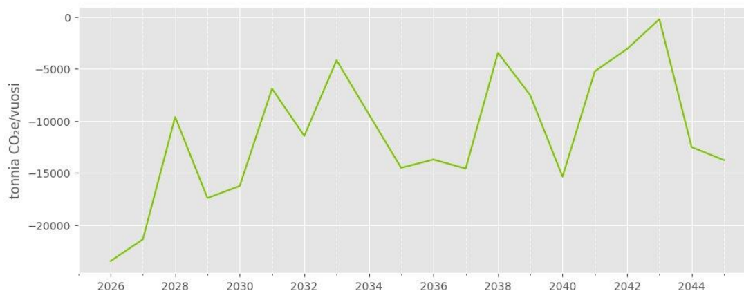
Bild 2: Lovisa stads skogars kolsänkor 2025–2045. Bilden visar hur mycket kol (koldioxidekvivalenter) Lovisa stads skogar binder eller frigör årligen 2025–2045 (i tusen ton CO 2 e/a). Ett negativt tal innebär att skogarna binder kol från atmosfären, ett positivt tal innebär att skogarna är en utsläppskälla. Storleken på skogarnas kolsänka varierar år från år, bland annat på grund av avverkningar. Andra orsaker kan vara väderförhållanden under året, plötsliga störningar (bränder, skadeinsekter med mera) samt skogarna åldersstruktur. Diagrammet visar dock att skogarna fortsätter att vara kolsänkor under hela den granskade perioden. I kolsänkornas storlek har man beaktat kol bundet i såväl trädbeståndet som i markgrunden.
