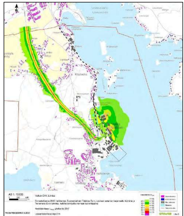
Bild 4.13. Bullerkällor i prognossituationen 2040, medelljudnivå LAeq, dagtid kl. 07–22 och nattetid kl. 22–07, bullerskydd byggda. Hamnens verksamhet har utvidgats och delvis flyttats till den västra sidan av banan.
