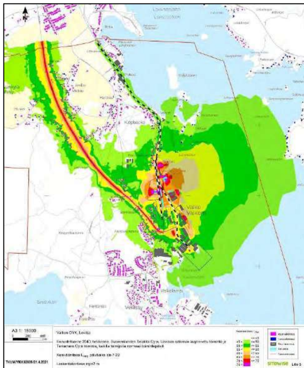
Kuva 4.13, Ennustetilanteen 2040 mukaiset melulähteet, keskiäänitaso LAeq, päiväaika klo 7–22 ja yöaika klo 22–7, meluesteet toteutettu. Sataman toiminta on laajentunut siirtynyt osittain myös radan länsipuolelle.
