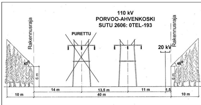
Tvärnsnitt av kraftledningen på 110 kV Borgå–Abborfors (2606) på detaljplaneområdet
