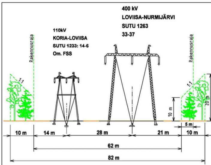
Tvärnsnitt av Fingrids kraftledning på 400 kV Lovisa–Andersböle (1263) och Carunas kraftledning på 110 kV Korja–Lovisa (1233) på detaljplaneområdet
