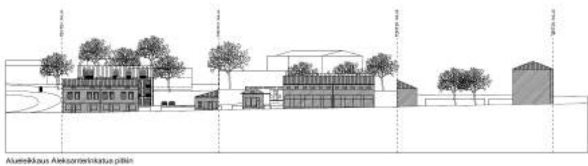
Kuva 6-4. Viitesuunnitelman alueleikkaus Aleksanterinkatua pitkin (Arkkitehtitoimisto Iiro Mikkola 2025).
