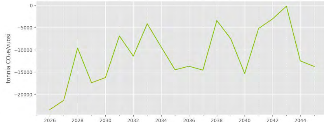
Kuva 4: Loviisan metsien hiilinielut 2025-2045. Arvion mukaan kaupungin metsät pysyvät hiilinieluna koko tarkasteluajan eli ne sitovat enemmän hiiltä kuin päästävät. (Sitowise, Loviisan metsien hiiliraportti 2025)
