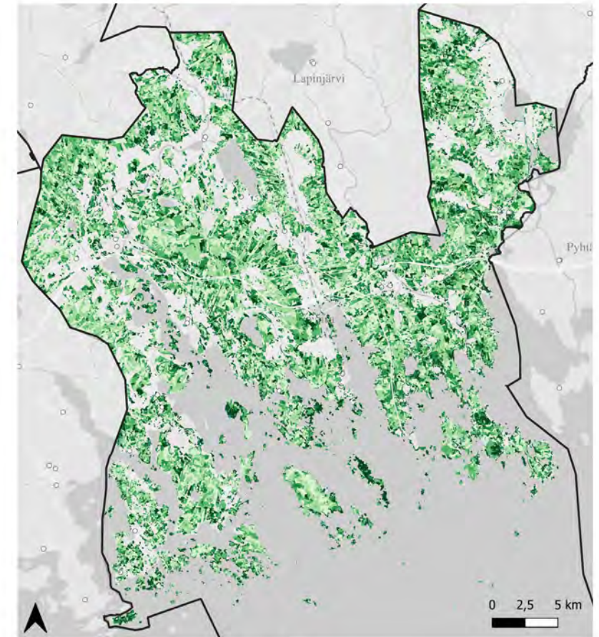
Loviisan metsien monimuotoisuus 2035
