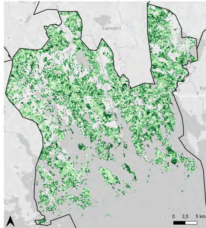
Loviisan metsien monimuotoisuus 2025
