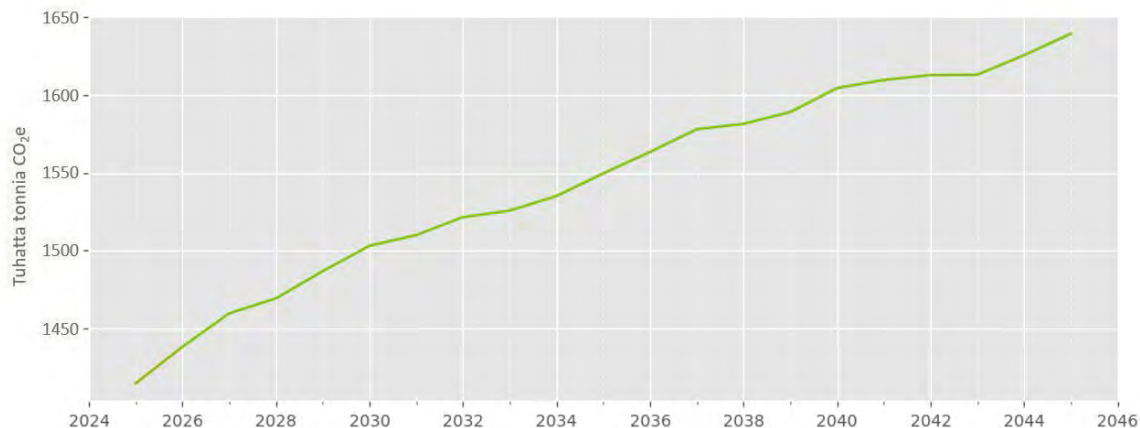
Kuva 3: Loviisan kaupungin metsien hiilivaraston arvioitu kehitys vuoteen 2045 saakka. Metsiin varastoituneen hiilen määrä kasvaa tasaisesti.
