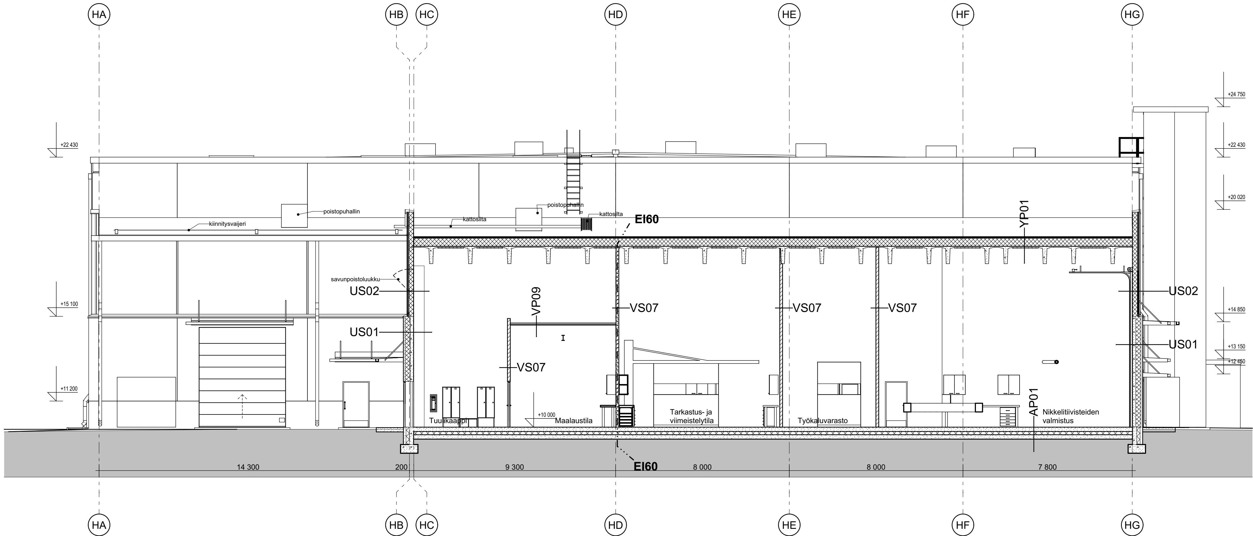
Kantavat rakenteet ja rakennetyypit RAK-suunnitelman mukaan
