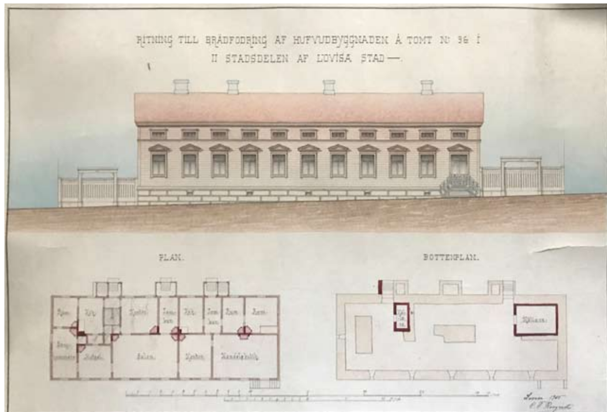
Tontti 36 päärakennus vuodelle 1905 päivätyn suunnitelman mukaan.
