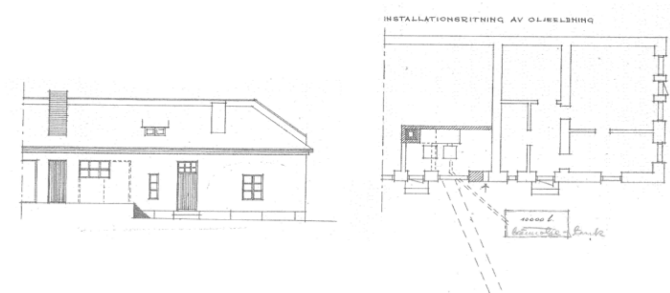
Rakennus R6, muutospirustus vuodelta 1962 / uusi pannuhuone ja savupiippu.
