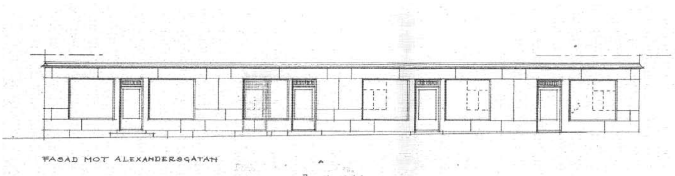
Tontti 37, päärakennus R5 muutospirustus katutason liiketilojen sisäänkäynneistä ja uusista näyteikkunoista 1962.
