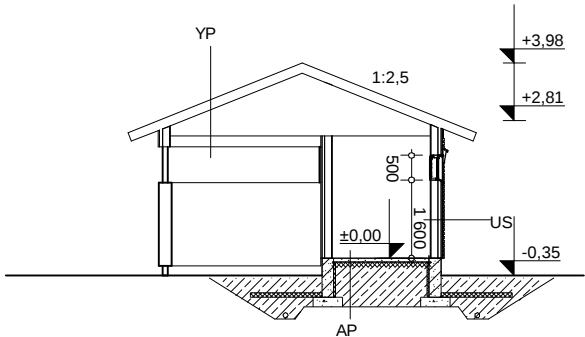
LEIKAUS B-B
