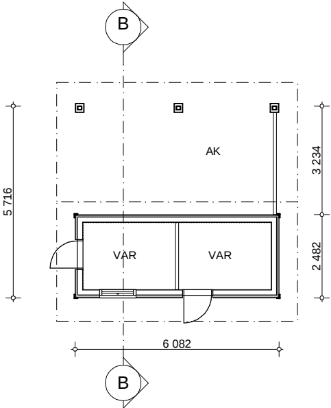
POHJAPIIRROS 1:100
